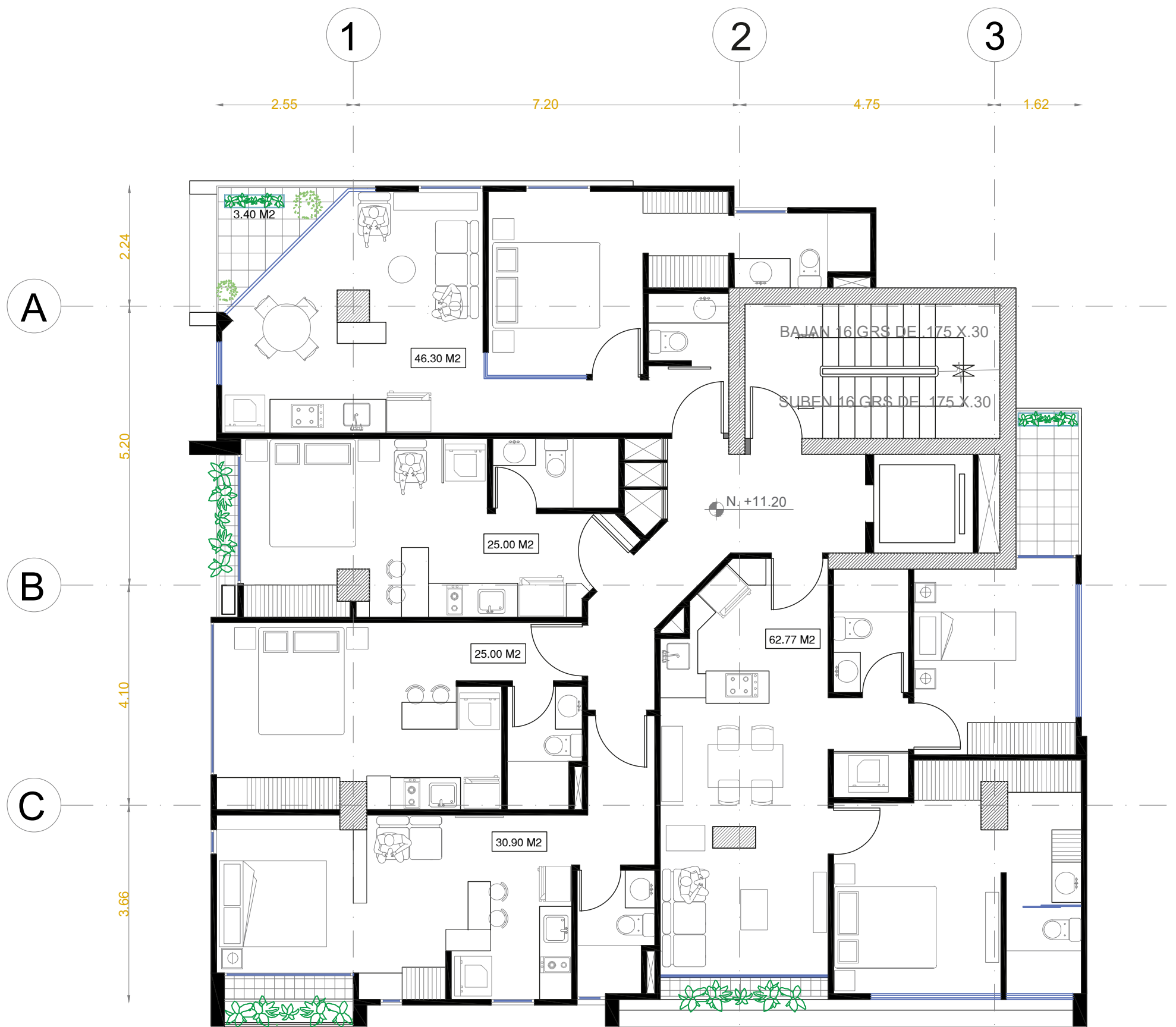
PISO 4 PLANTA NIVEL +11.20 1 SUITE + 3 ESTUDIOS + 1 DEPTO. TIPO 2
